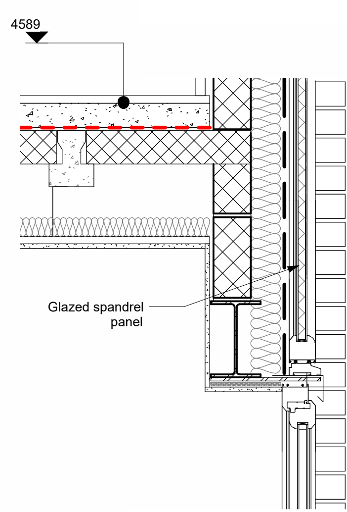
Detail 1 1 : 10
