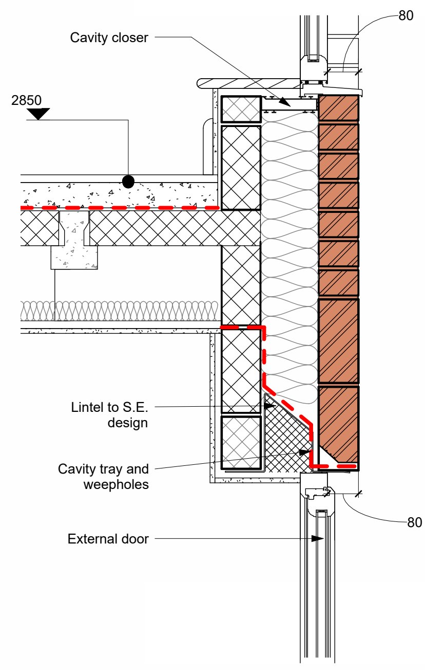
Detail 2 1 : 10
