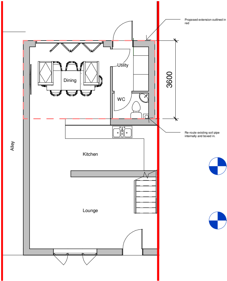
Prop. Grund Floor Plan 1 : 100
